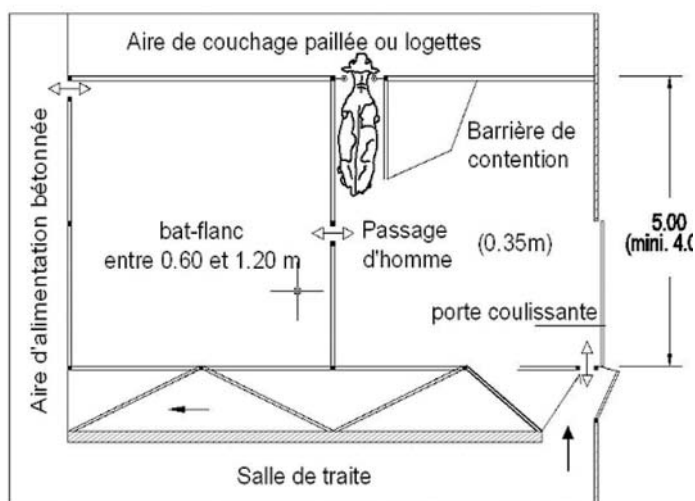
Aménagement d'un box vêlage (source GIE Bretagne)
