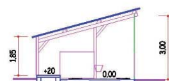
Coupe de Principe
