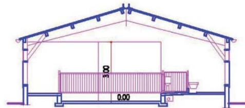
Coupe de Principe
