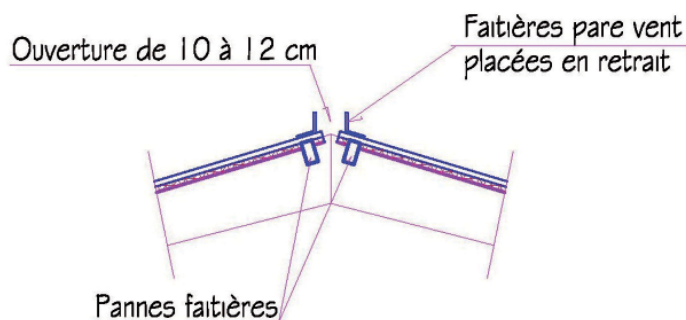
Schéma de principe d'un faitage ouvert
